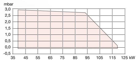
CURVA DE FUNCIONAMIENTO Quemador BENTONE ST146 KS
